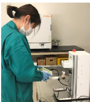
食感試験装置のレオメーター。市田柿を測定中
